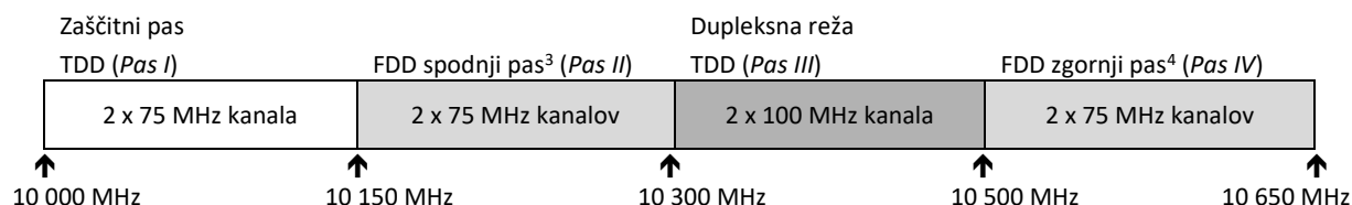
Slika 1: 10 GHz pas
