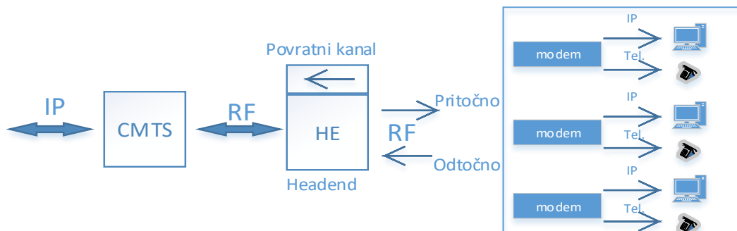
Slika 9: Shema kablanskega omrežja
