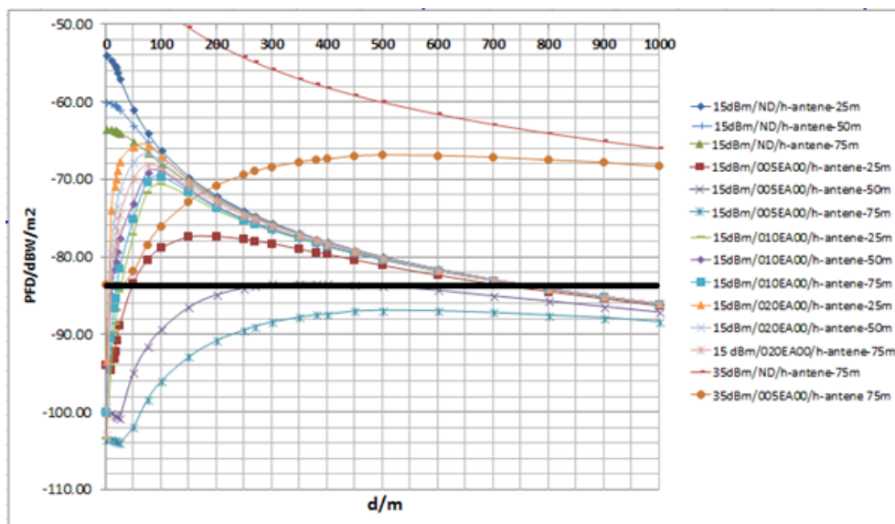
Slika 14: Porazdelitev gostote pretoka moči (PFD) v odvisnosti od višine antenskega stolpa in sevalnega diagrama oddajne antene 31 (EIRP = 15 dBm, h = 25, 50 in 75 m)
