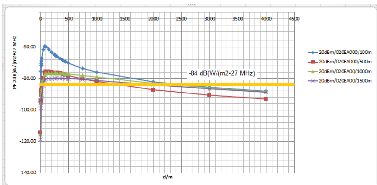
Slika 18: Separacijska razdalja med oddajnikom MMDS in satelitskimi sprejemniki pri efektivni izsevani moči (EIRP) 20 dBm za različne višine oddajne antene nad okoliškim terenom ( h = 100, 500, 1000 in 1500 m)
